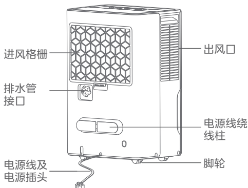
除湿机背面
